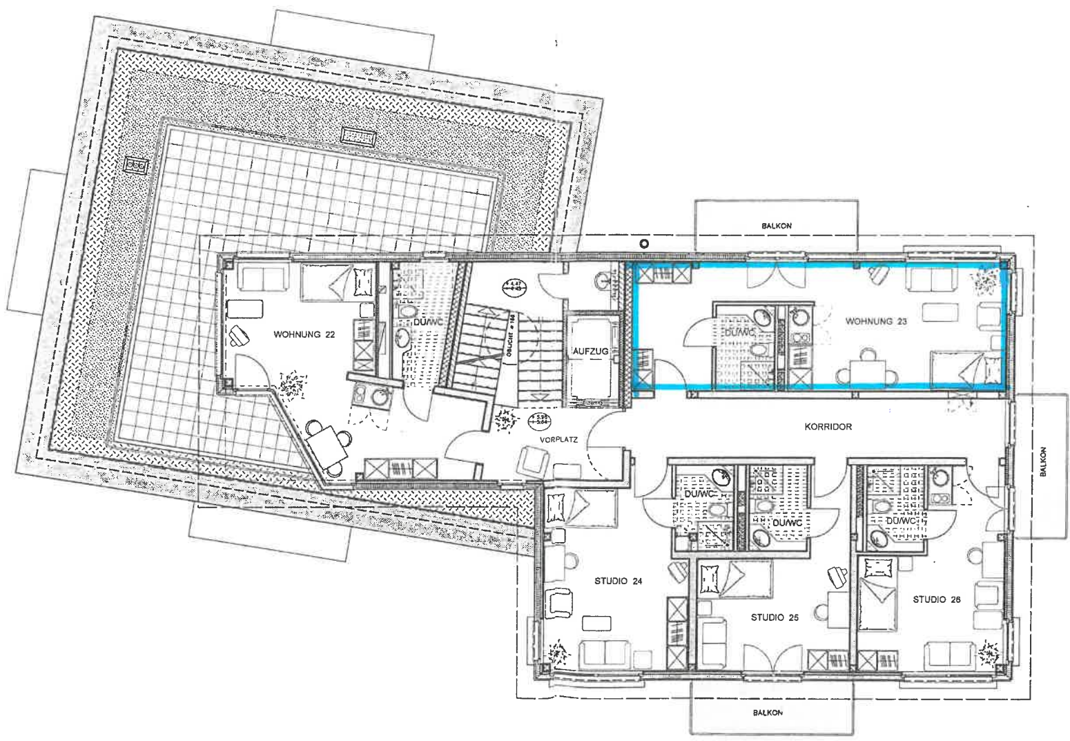
NEUBAU : ATTIKAGESCHOSS GRUNDRISS 1: 100
