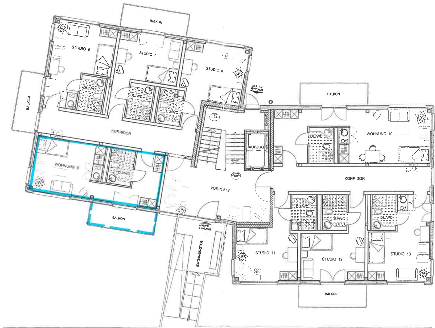
NEUBAU : ERDGESCHOSS GRUNDRISS 1: 100
