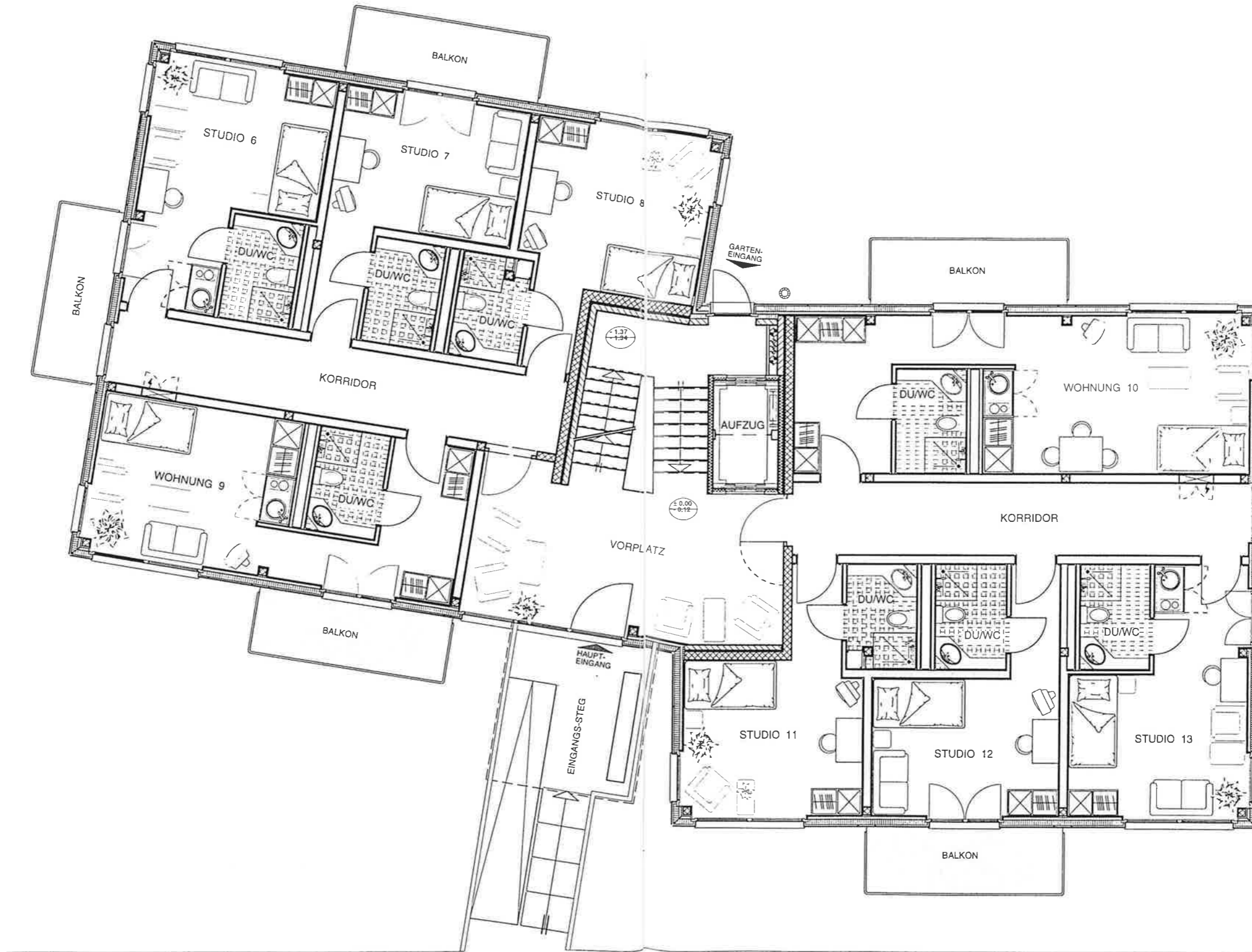
NEUBAU : ERDGESCHOSS GRUNDRISS 1: 100
